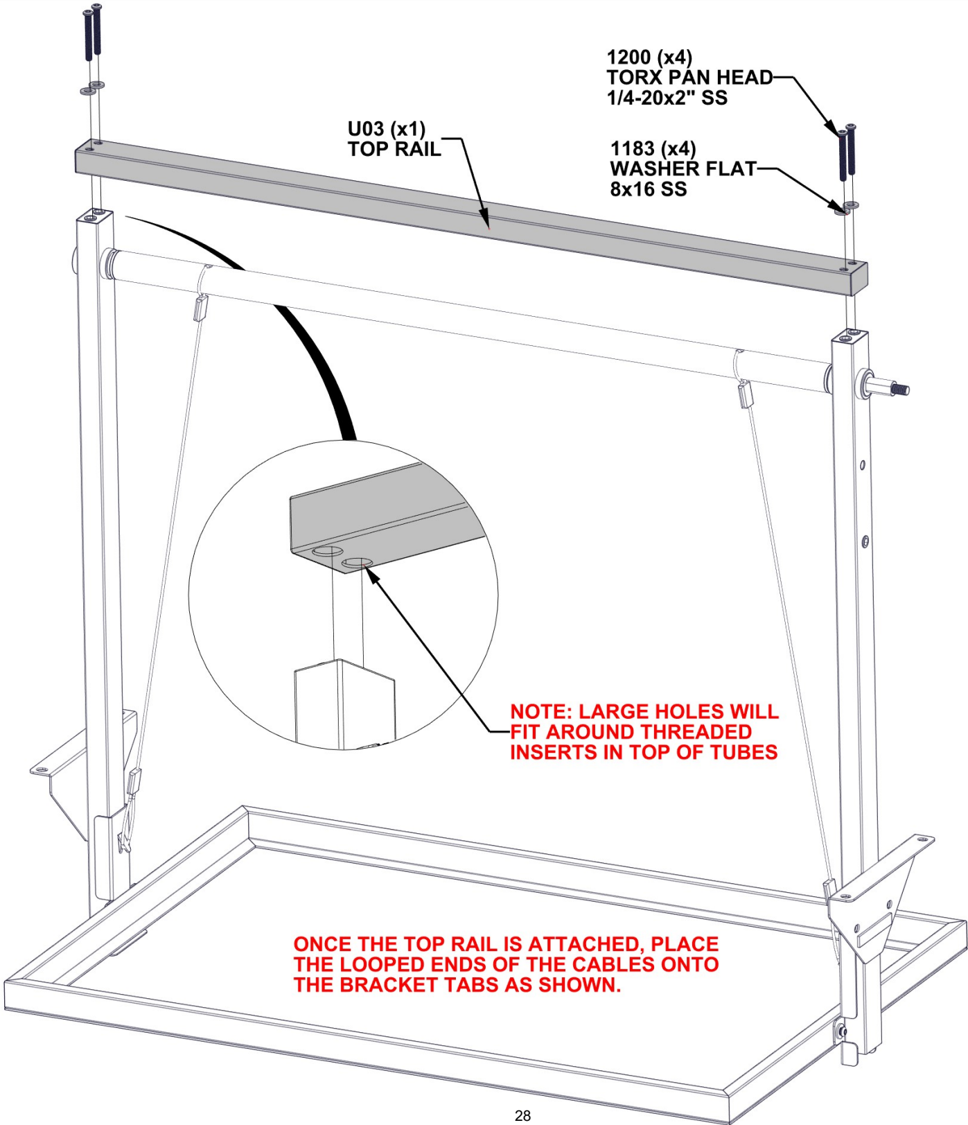
U03 TOP RAIL - A4M02149 (x1) 1"x1 1/2"x35 1/4" (25x38x896)
