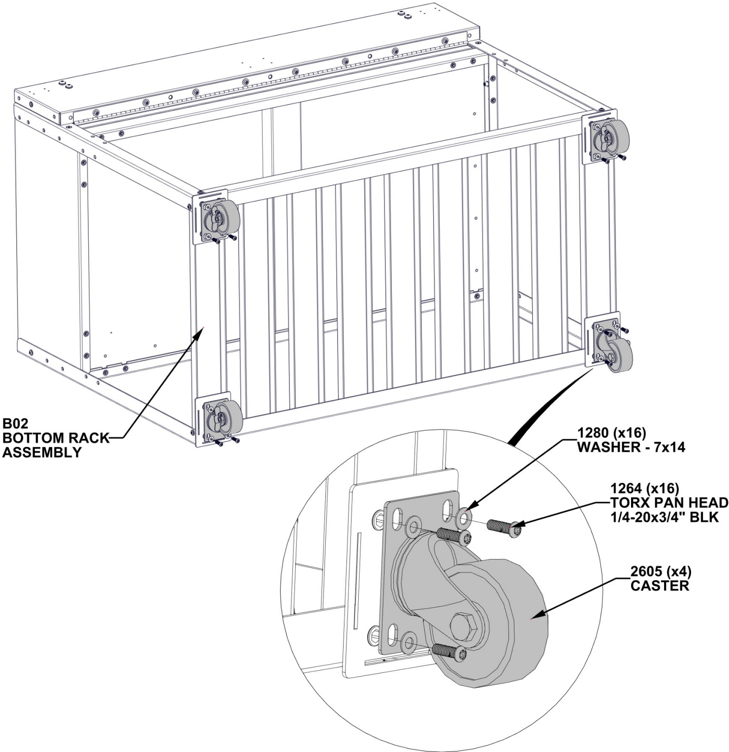
A4M02605 CASTER (x4)
