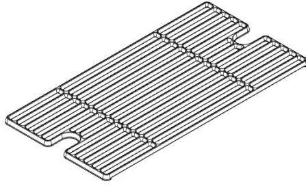
G02 GRATE - A4M02145 (x3) 7/16"x10 1/2"x20 1/2" (12x266x520)
