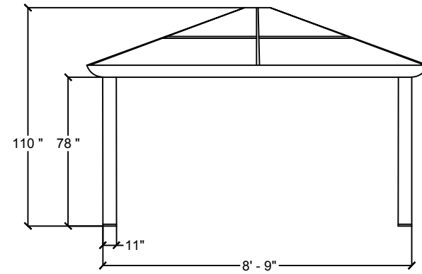
VUE DE CÔTÉ (LARGEUR) SIDE VIEW (WIDTH)
