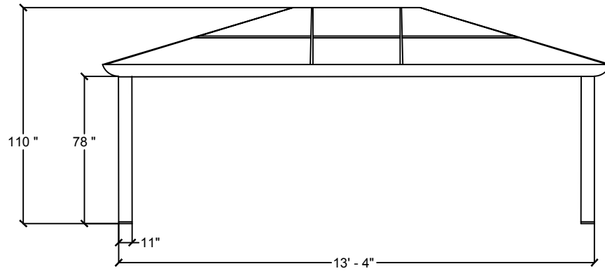
VUE DE CÔTÉ (LONGUEUR) SIDE VIEW (LENGTH)
