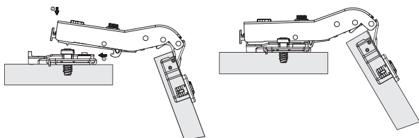
Bisagra de 45°
