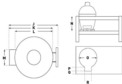
OBENSICHT
