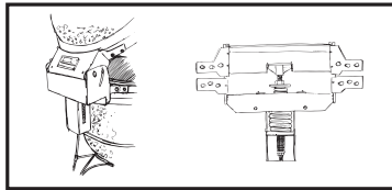
BISAGRA ALTERNATIVA
