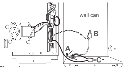
Figure 4 120 Volt
