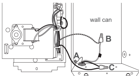
Figure 3 240 Volt
