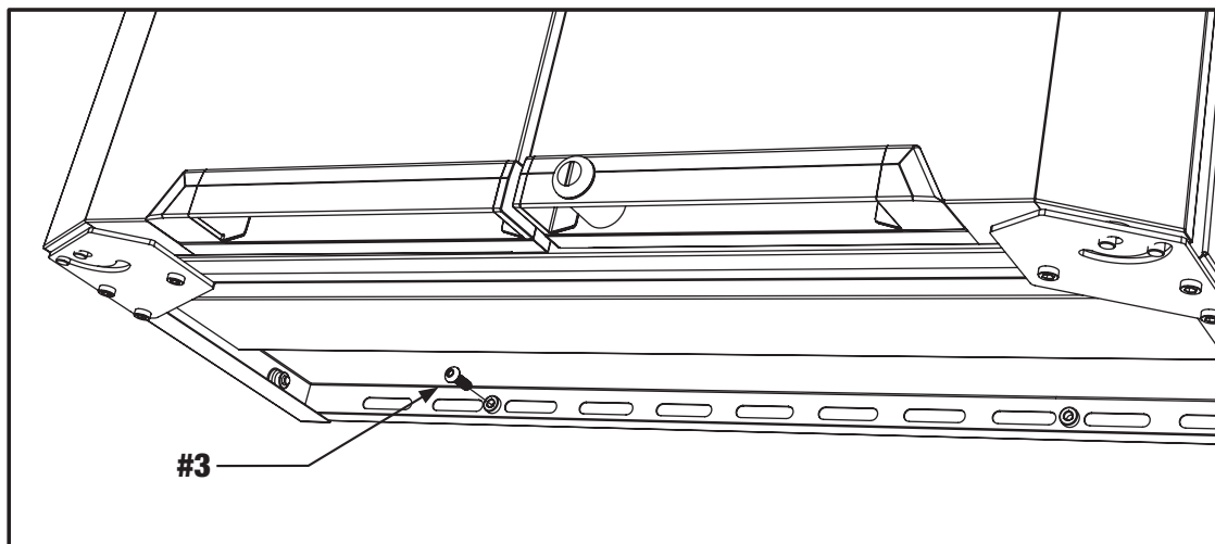
INSERTAR EL TORNILLO DEL LADO DE LA PUERTA COLGANTE INFERIOR
