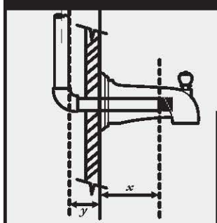
Instalación del surtidor de la tina
