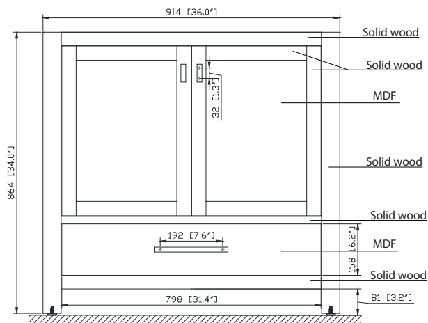
Front / Devant
