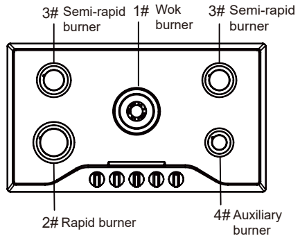
PRO GH2365SF/PRO GH3365SF
