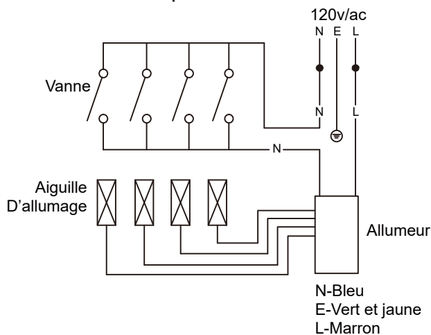
PRO GH2304SS/PRO GH2304SF
