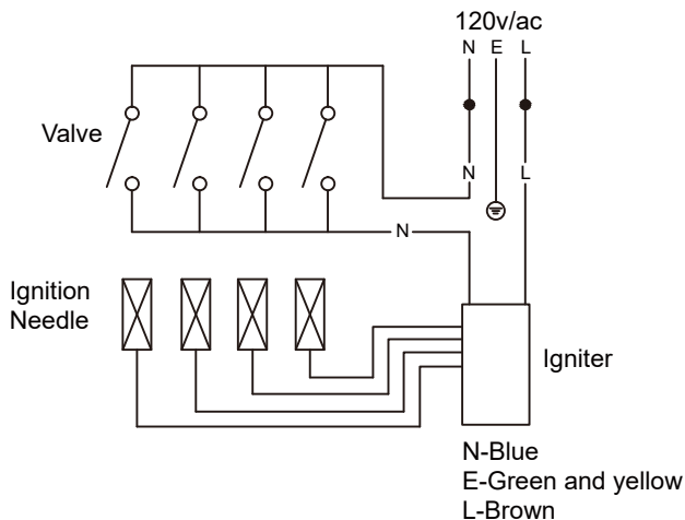
PRO GH2304SS/PRO GH2304SF
