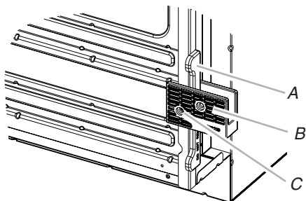
A. Separador B. Pata C. Tornillo n.º 8-18 x 3/8" (9,5 mm)
