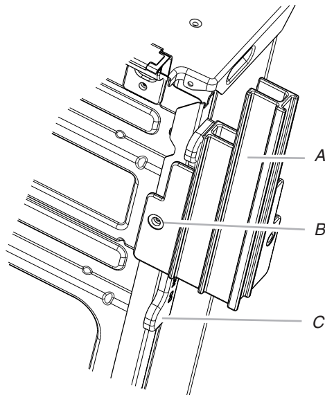
A. Pata delantera B. Tornillo n.º 8-18 x 3/8" (9,5 mm) C. Separador
