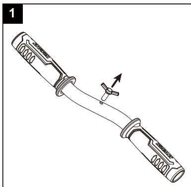
Unscrew wing nut.
