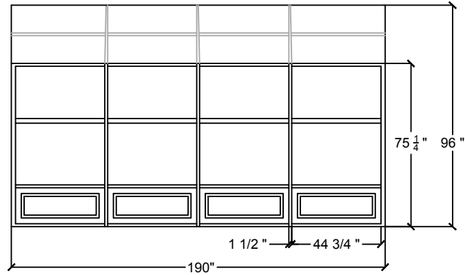
VUE DE CÔTÉ (LONGUEUR) SIDE VIEW (LENGTH)
