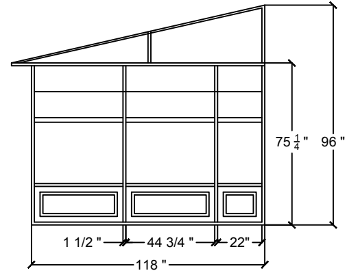
VUE DE CÔTÉ (LARGEUR) SIDE VIEW (WIDTH)
