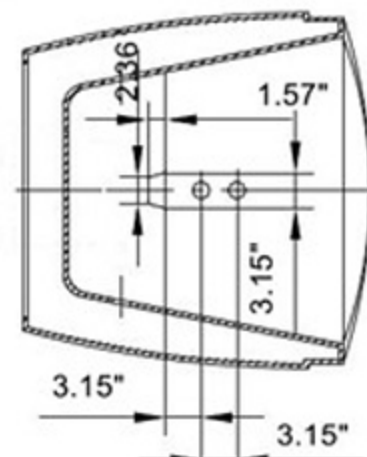
B2-B2
