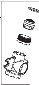
RP102039 1.2 GPM (4.5 L/Min) Aerator & Wrench Aireador y Llave Aérateur et Clé
