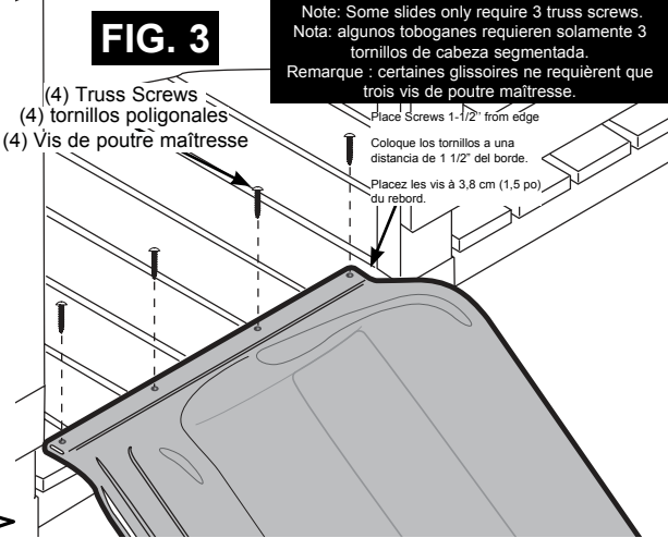
(4) 1" Truss Screw Vis de poutre maîtresse de 1 po (25 mm) Tornillos poligonales de 1" (2.5 cm)
