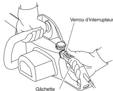
Figure 10 - Emplacement du bouton de verrouillage et de la gâchette
