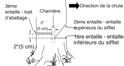
Figure 12 - Abattage d'un arbre
