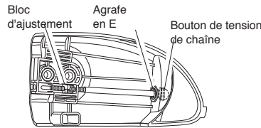
Figure 6- Tournez la vis de tension de chaîne sur les modèles RM1635W
