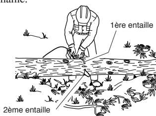
Figure 16 - Tronçonnage d'une bille soutenue aux deux extrémités
