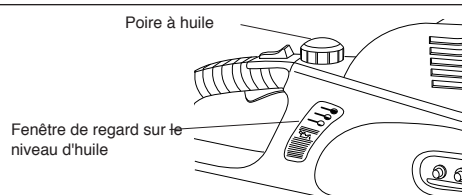
Figure 7 - Emplacement de la poire à huile et de la fenêtre de regard sur le niveau d'huile pour le modèle RM1632A
