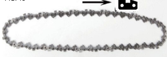
FIG. 13 Direction de la chaîne
