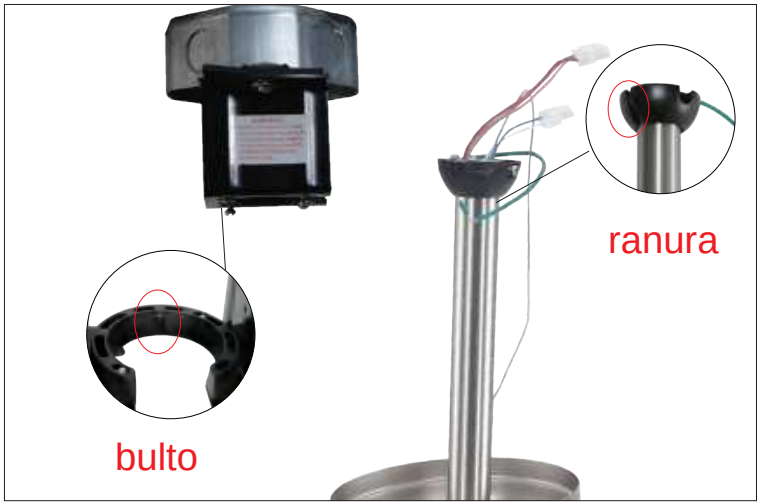
Paso 10 Cuelgue el ventilador en el soporte de suspensión de modo que los salientes del soporte de suspensión queden alineados con las muescas de la semiesfera.
