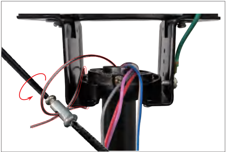
Paso 11 Instalación de cuerdas de Seguridad.
