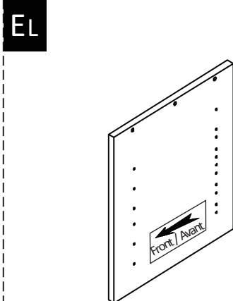
LEFT DIVIDER QTY 1
