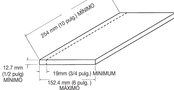
41 DIMENSIONES QUE ACEPILLAN DEL MÍNIMO Y DEL MÁXIMO
