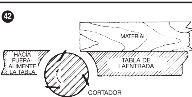
ALIMENTACION INDEBIDA - A CONTRAHILO
