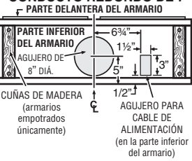
CONDUCTO REDONDO DE 7"
