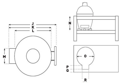
OBENANSICHT
