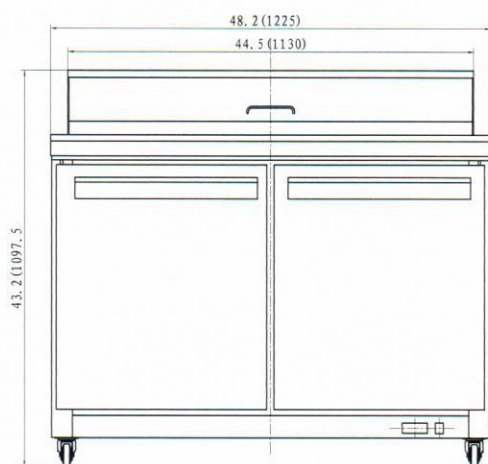
MXCR-48S
