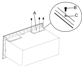
A. Conduit de refroidissement côté gauche B. Vis cruciformes (3) C. Trous de vis (3)
