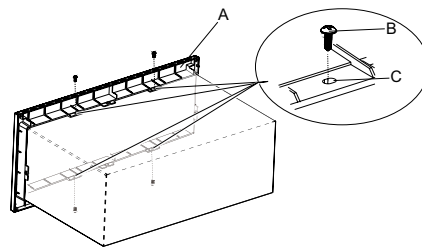
A. Cadre de garniture B. Vis à tête à tête ronde n° 7-18x7/16 po (4) C. Trous de vis (4)
