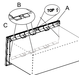
A. Cadre de garniture B. Goupille de positionnement (4) C. Fente de positionnement (4)
