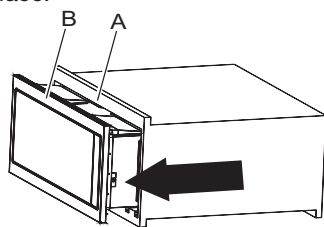
A. Armoire B. Four à micro-ondes
