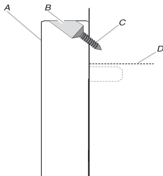
A. Cadre de garniture B. Rail de guidage du trou de montage C. Vis à bois à tête plate n° 7-16x15/16 po (4) D. Plafond de l'ouverture d'encastrement
