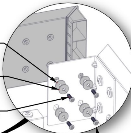
040 (x16) BOLT - M6x20
