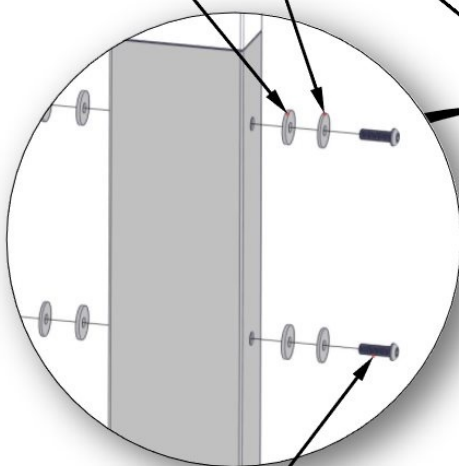
040 (x4) BOLT - M6x20
