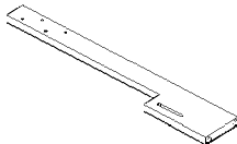
x1 RD364-230-1-LEGR Headboard legs (right) * Pattes de la tete de lit (droite) Pattes de cabecera (derecha)
