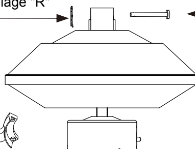
Assemblage ventilateur-moteur
