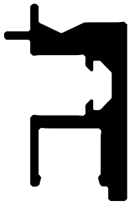
Linteau (Qté 1)
