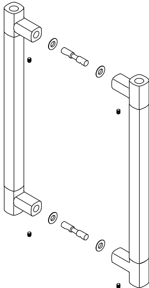
Poignée (Qté 1)
