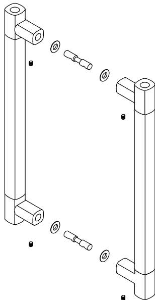
Manija (cant. 1)
