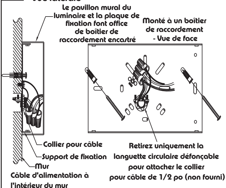
B1 Monté sans boîtier de raccordement - Vue latérale
