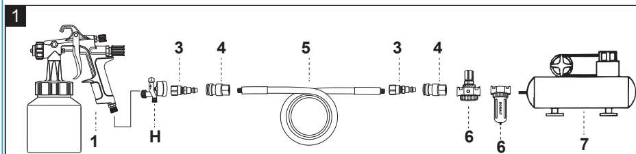
Montage recommandé de la conduite d'air
