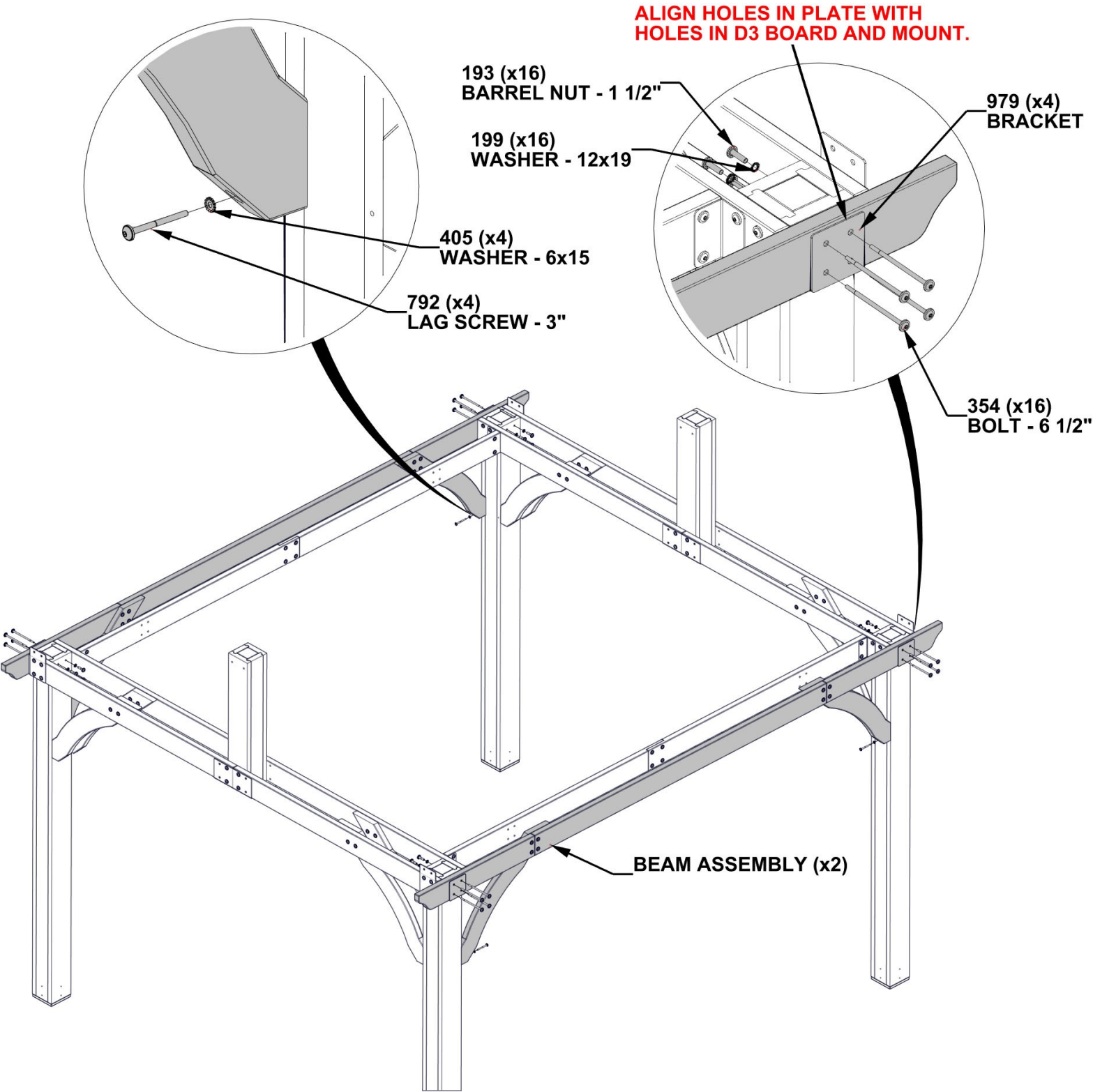
A4M00979 (x4) BRACKET
