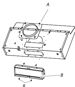
Installez les raccords de transition rectangulaire 8,3 x 25,4 cm (3¼ x 10 po) A. 8,3 x 25,4 cm (3¼ x 10 po)
