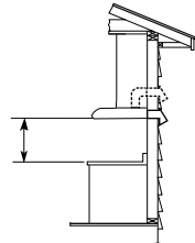
Ventilation à travers le mur
