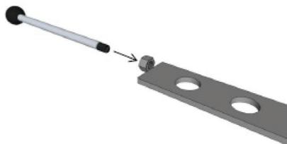
Figure 2 Installation de la tige de commande d'air supérieure
