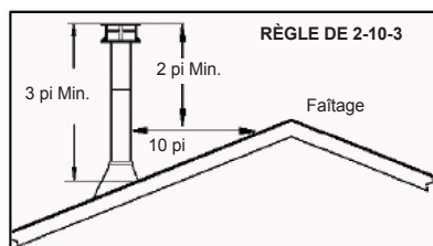
Figure 8 Exigences relatives à la hauteur de la cheminée
