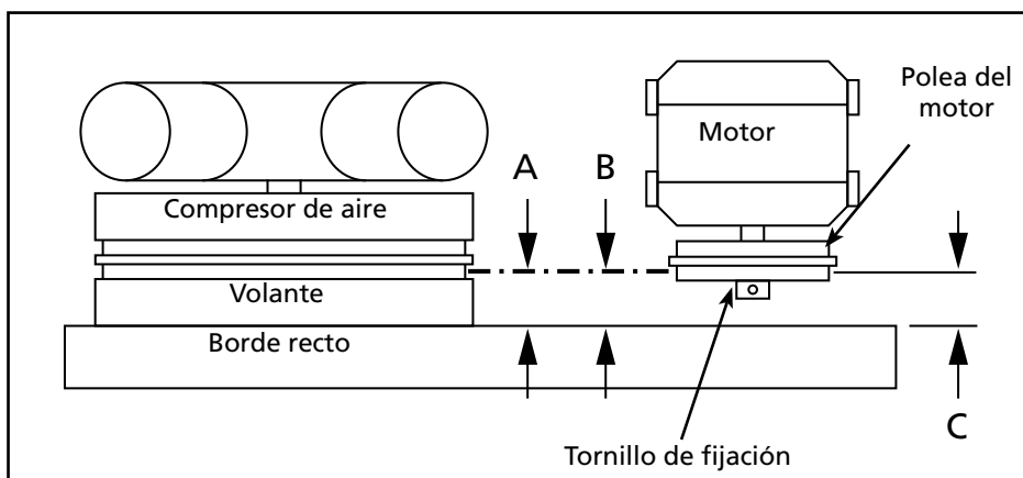
Figura 20 - Vista superior
