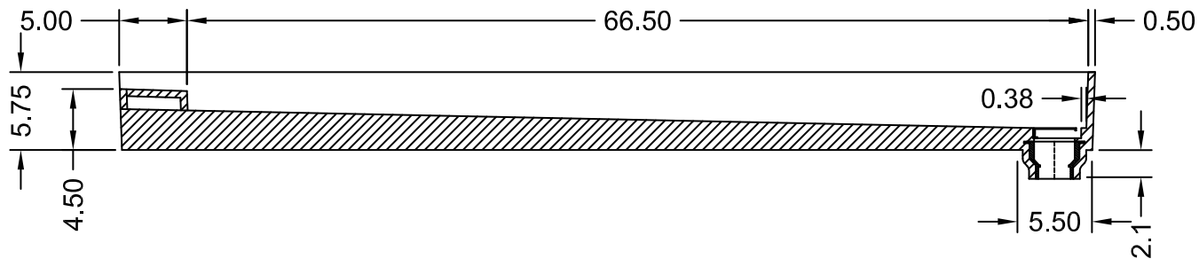
SECTION A-A
