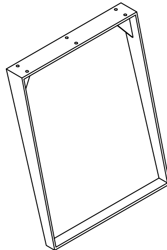
LEG QTY 2
