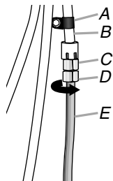
A. Abrazadera en "P" B. Línea de agua de plástico C. Puerto de entrada de la válvula de agua D. Tuerca de compresión E. Tubería de cobre
