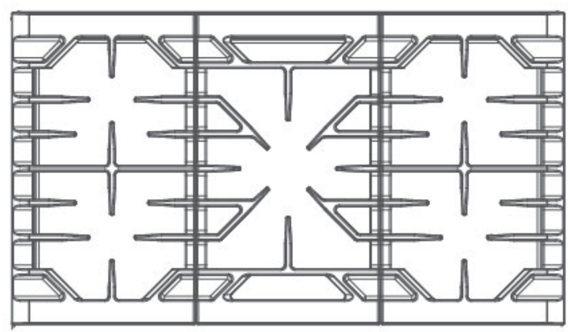
锅支架（3）
