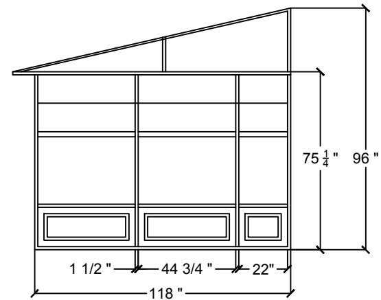
VUE DE CÔTÉ (LARGEUR) SIDE VIEW (WIDTH)
