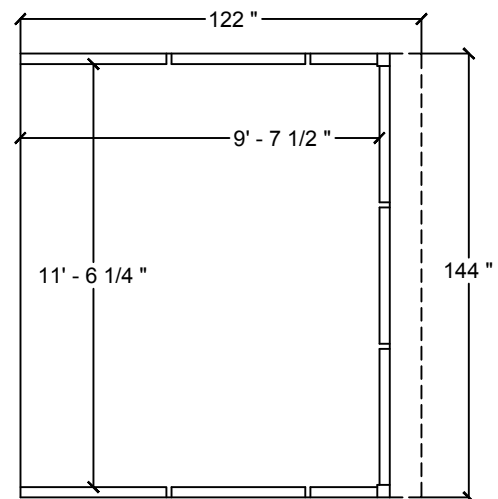
REBORD DU TOIT ROOF OVERHANG
