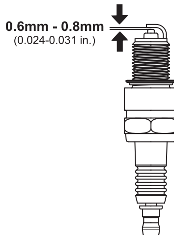
Vérifier l'écart des bougies
