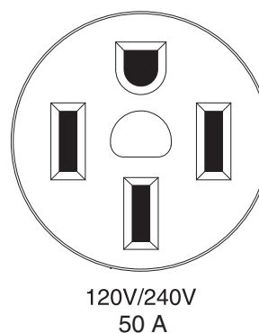
Figura 8 - Receptáculo de 120/240 VAC, 50 Amp
