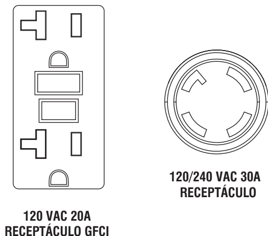
Figura 6 – Receptáculos del generador
