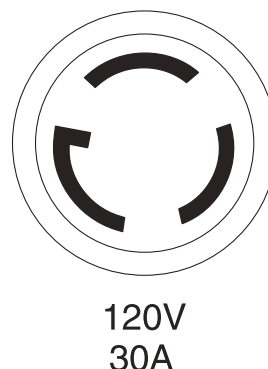
Figura 7 - Receptáculo de 120 VAC, 30 Amp
