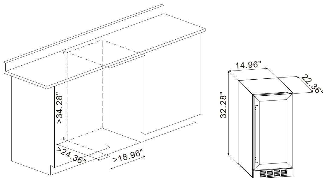
⊙ Schéma d'installation
