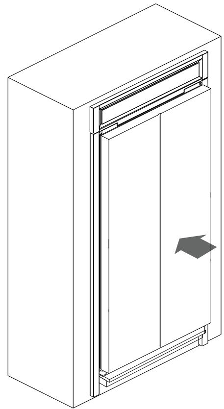
6 INSERT THE REFRIGERATOR INSÉREZ LE RÉFRIGÉRATEUR
