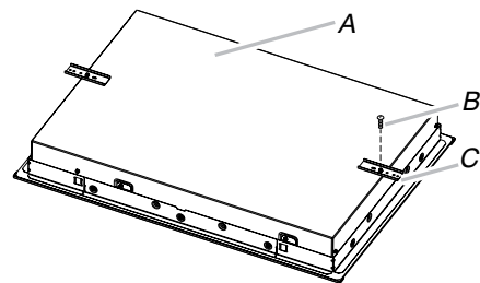
A. Partie inférieure de la base de la table de cuisson B. Vis d'attache C. Brides de fixation
