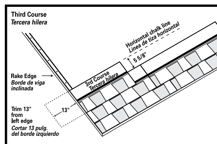
FIG 5C Shingle Application Instalación de las tejas
