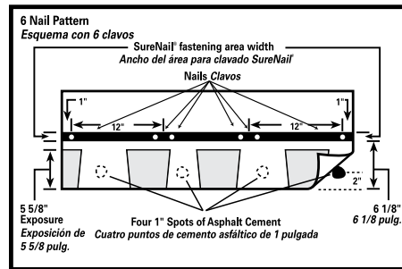
FIG 4B Mansard and Steep Slope Application Esquema de instalación en pendientes pronunciadas o mansardas
