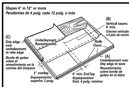
FIG 2 Underlayment Standard Slope Pendiente estándar del revestimiento
