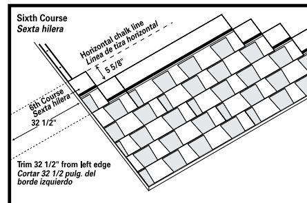
FIG 5F Shingle Application Instalación de las tejas
