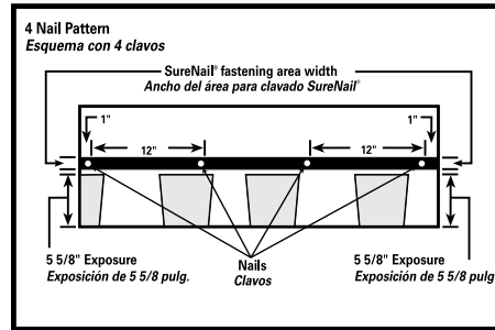
FIG 4 Standard Fastening Pattern Esquema de instalación estándar
