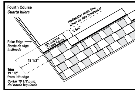
FIG 5D Shingle Application Instalación de las tejas
