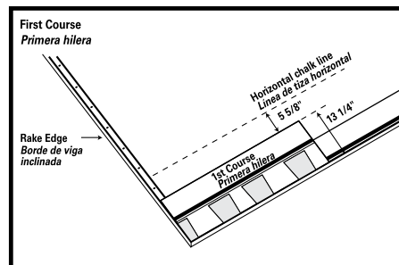
FIG 5A Shingle Application Instalación de las tejas
