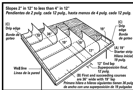
FIG 3 Underlayment Low Slope Pendiente baja del revestimiento
