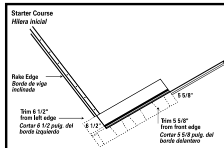
FIG 5 Shingle Application Instalación de las tejas
