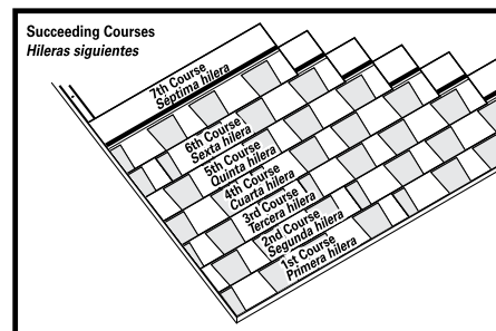
FIG 5G Shingle Application Instalación de las tejas
