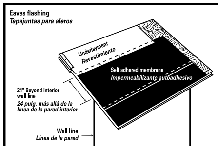
FIG 1 Specialty Eave Flashing Tapajuntas especial para aleros
