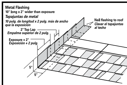
FIG 7 Step Flashing Tapajuntas escalonado
