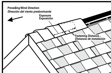
FIG 8 Hip & Ridge Application Aplicación para caballete y cumbrera
