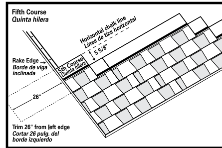
FIG 5E Shingle Application Instalación de las tejas
