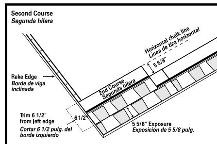
FIG 5B Shingle Application Instalación de las tejas
