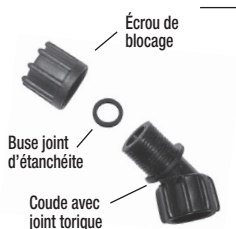
6-8148 Trousse de buse
