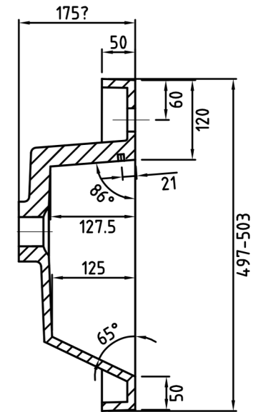
SECTION A-A
