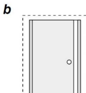
b FINITION DE CALES ET D'APLOMB MONTANT AVEC PORTE
