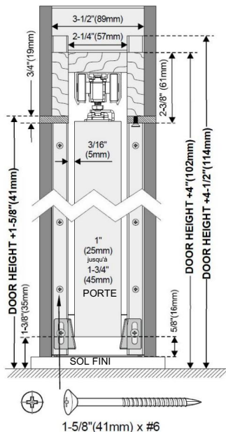
b FINITION DE CALES ET D'APLOMB MONTANT AVEC PORTE
