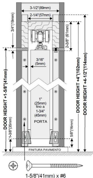
FINITURA A SPESSORE E A PIOMBO STIPITE CON PORTA
