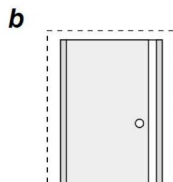
FINITURA A SPESSORE E A PIOMBO STIPITE CON PORTA
