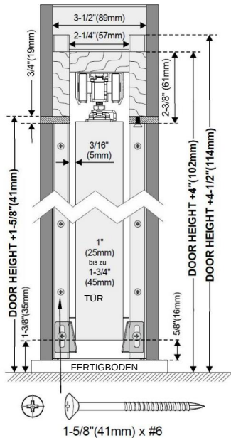
UNTERLEGSCHLEIBEN- UND LOT-FINISH Türpfosten mit Tür
