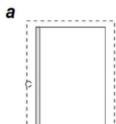
ATTACCO FINITURA SPLIT STIPITE A TUBO DI ACCIAIO/ PORTA A PIOMBO CON STIPITE
