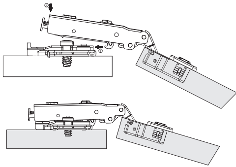
105° Hinge
