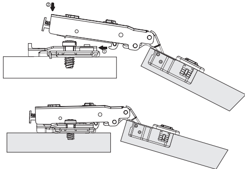
Bisagra de 105°
