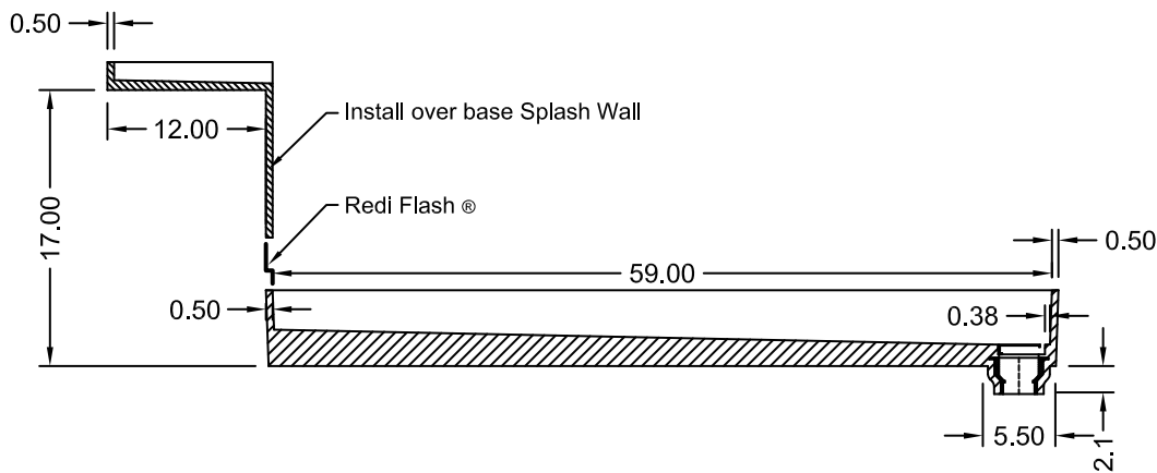
SECTION A-A
